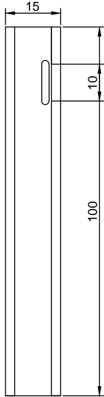
右視圖
