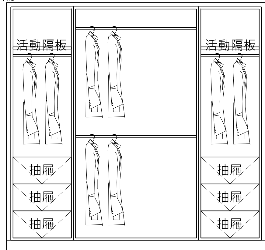
衣櫃詳細圖
