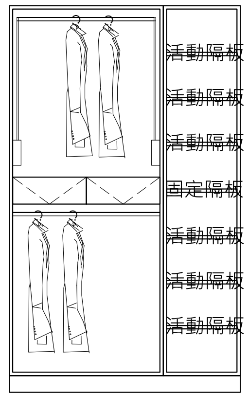
衣櫃詳細圖
