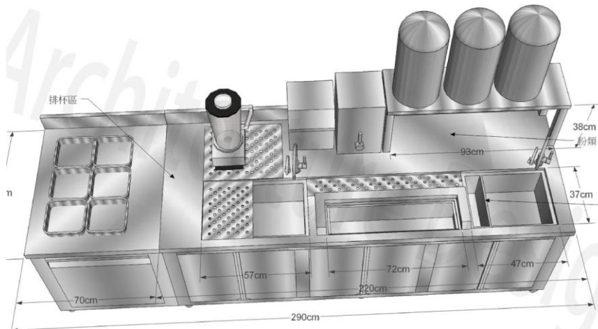
餐飲雪克台設計
