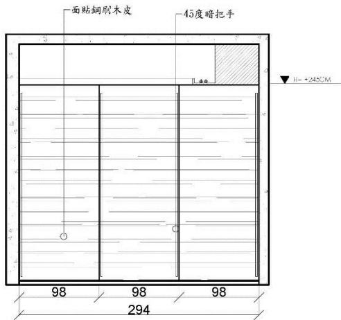
主臥室衣櫃面立面施工圖
