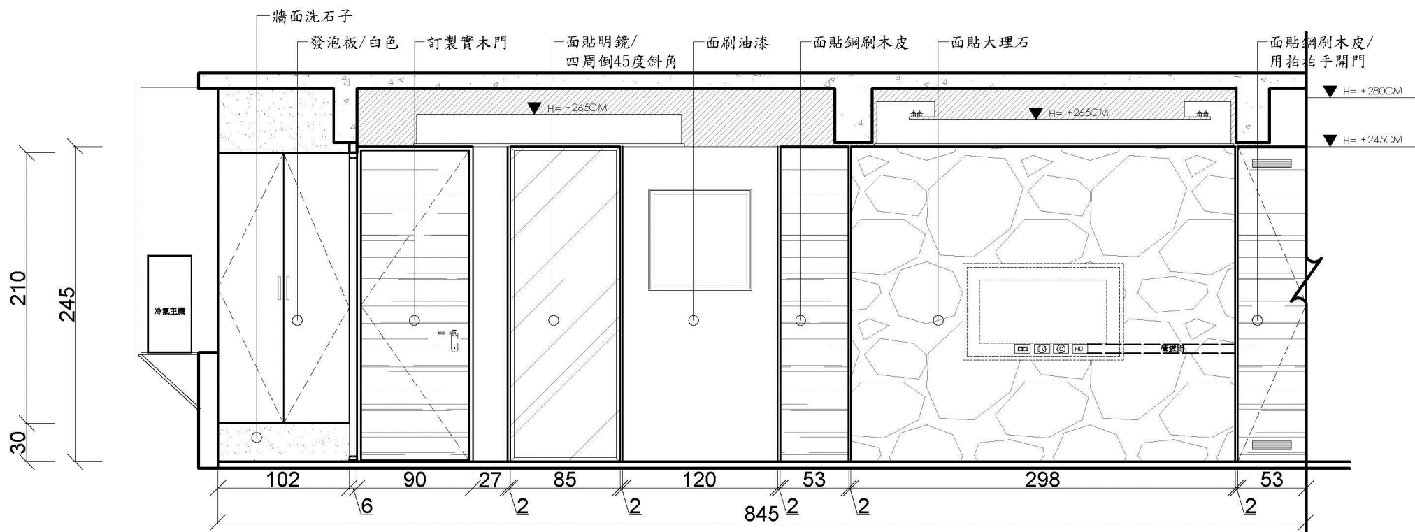
玄關及電視牆立面施工圖
