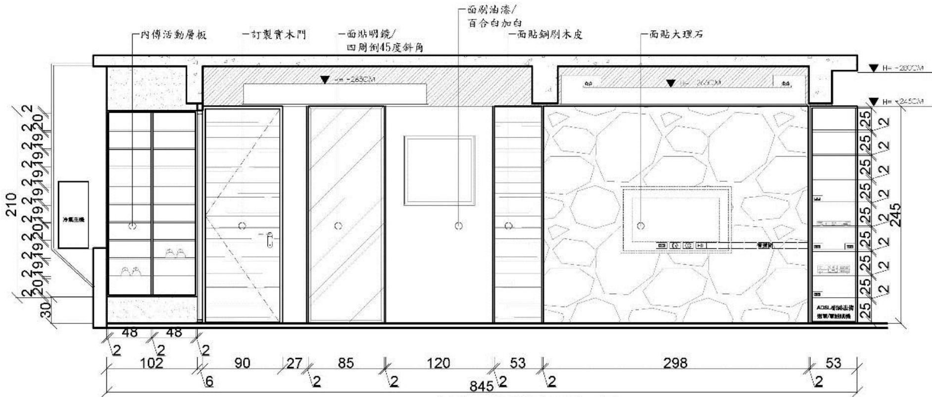
玄關及電視牆立面施工圖
