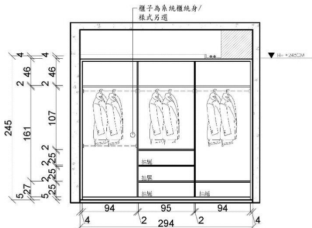
主臥室衣櫃面立面施工圖
