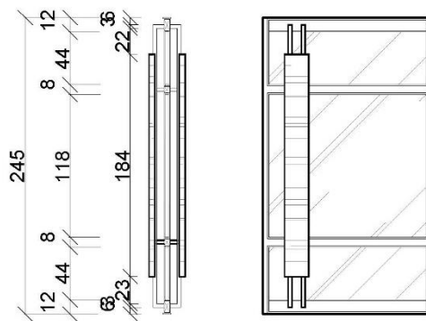
客/餐廳拉門立面施工圖
