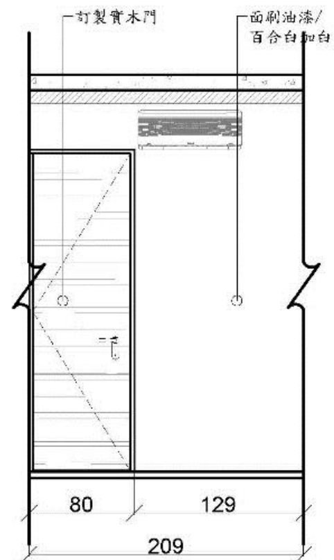
餐廳/浴廁立面施工圖
