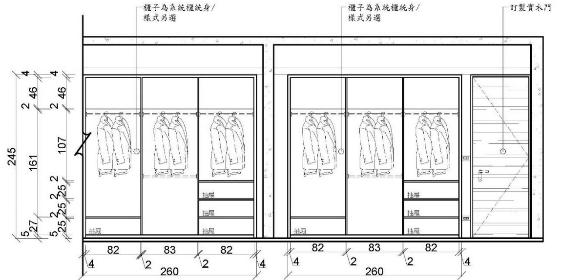
臥室一~二衣櫃面立面施工圖
