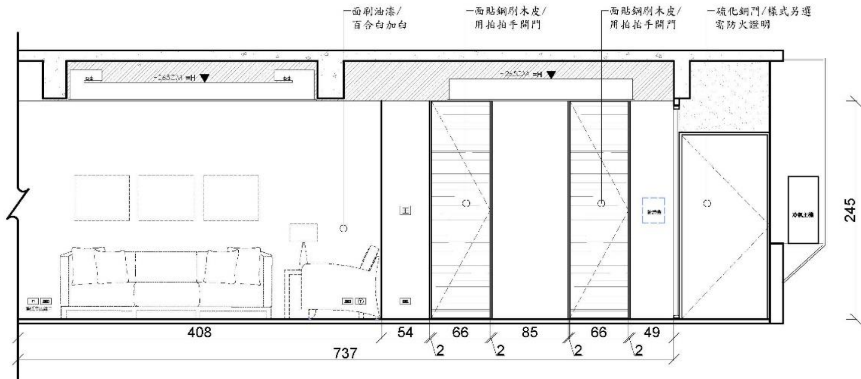
玄關及沙發背牆立面施工圖
