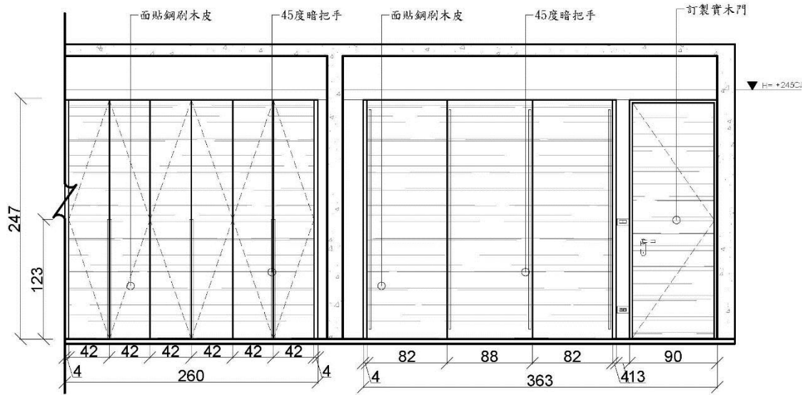
臥室一~二衣櫃面立面施工圖
