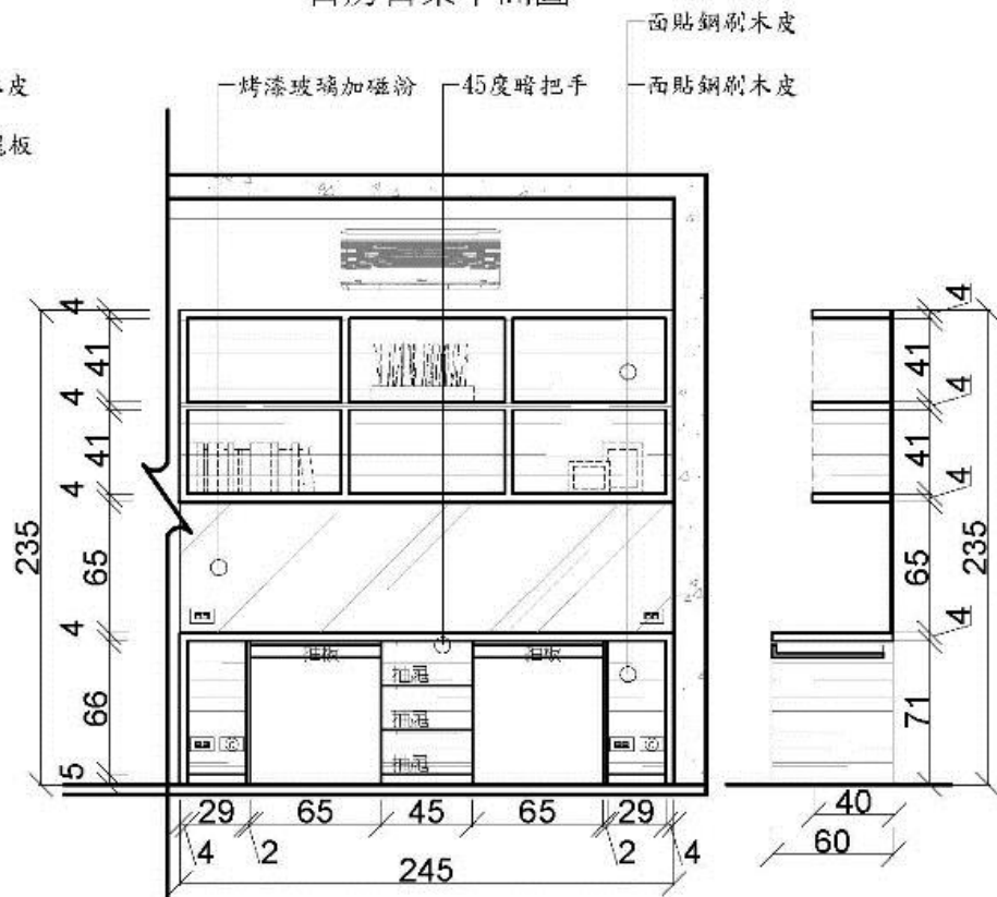
書房書桌立面施工圖
