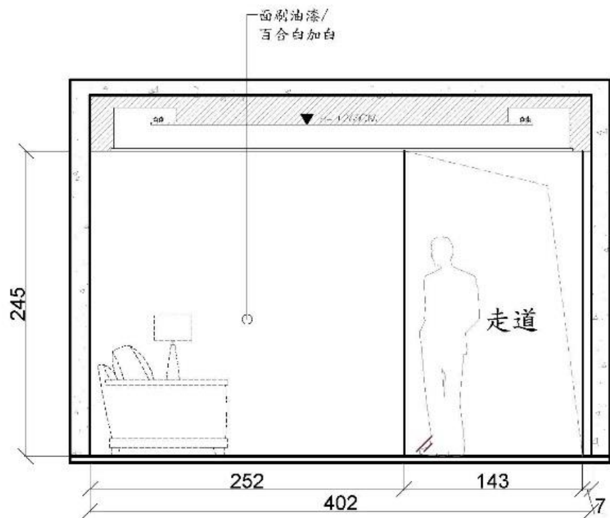
客廳左側立面施工圖
