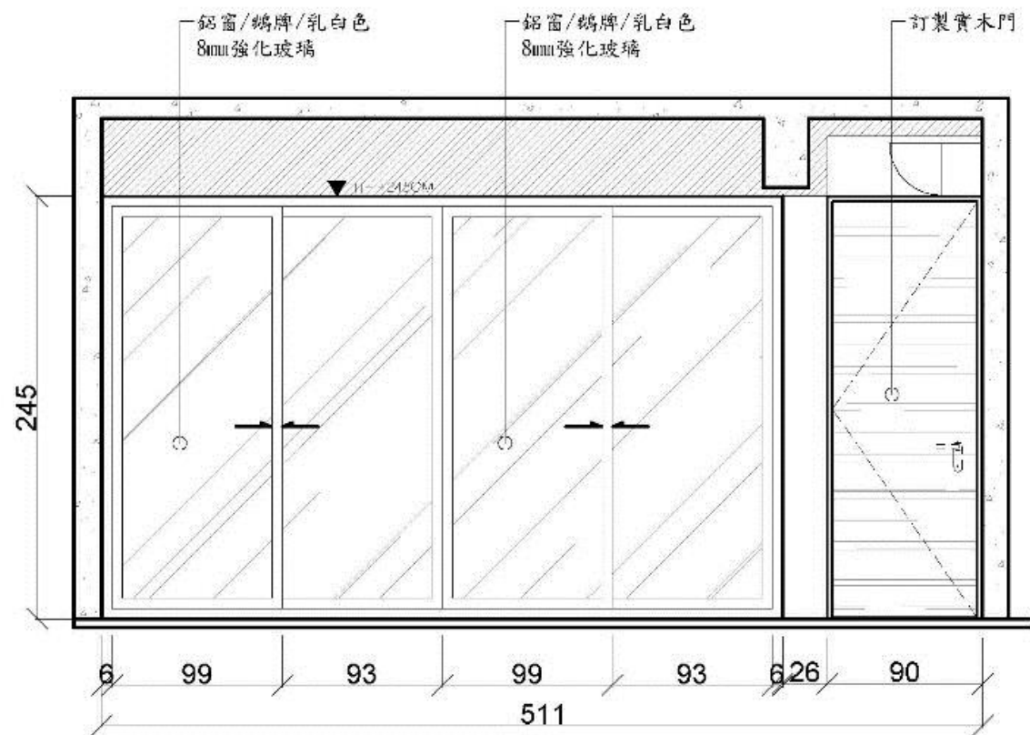
餐廳/戶外平台立面施工圖
