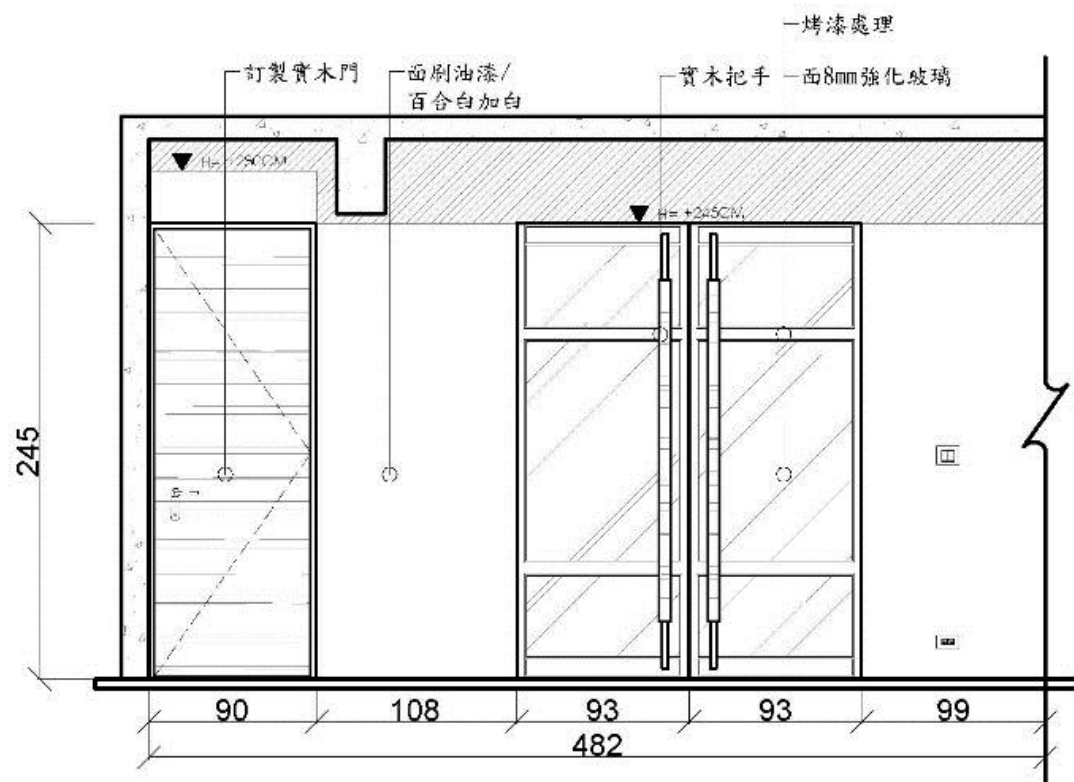
書房拉門立面施工圖
