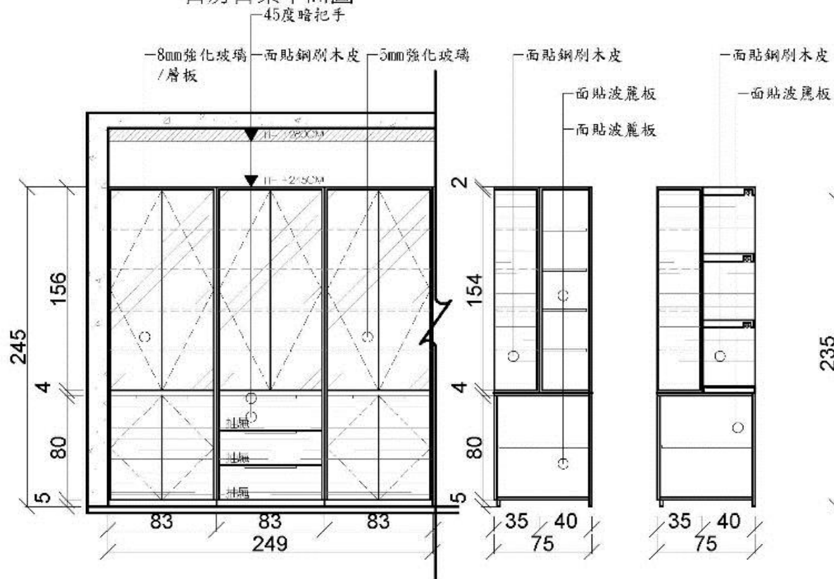
書房書桌立面施工圖
