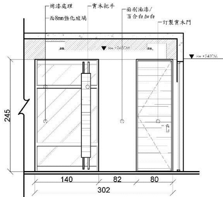
餐廳/客廳立面施工圖
