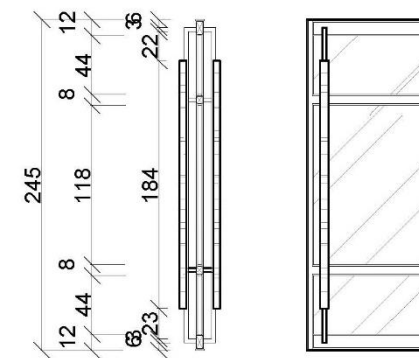
書房拉門立面施工圖
