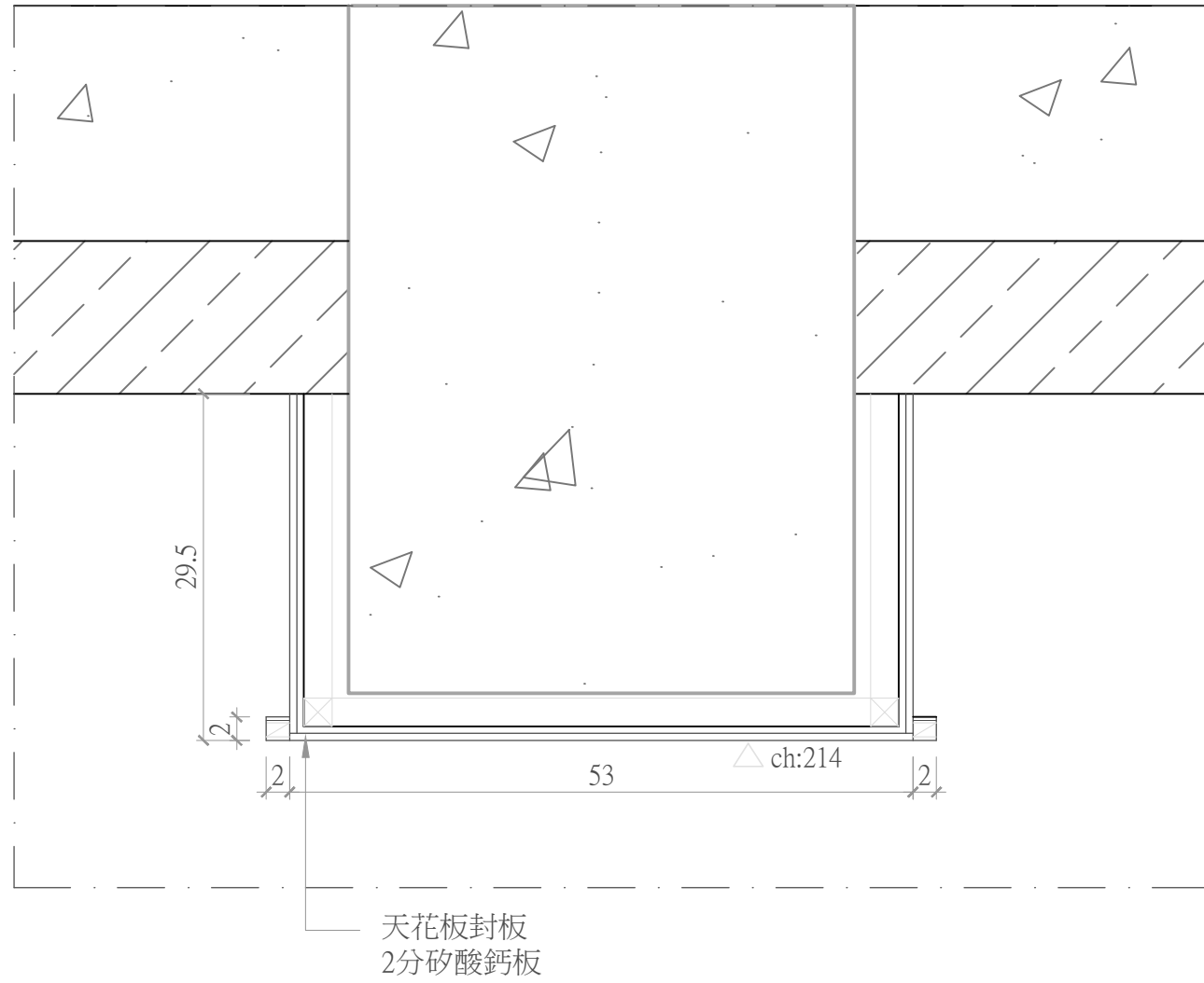
01 餐廳電視牆造型梁大樣圖 ID-01 S:1/60
