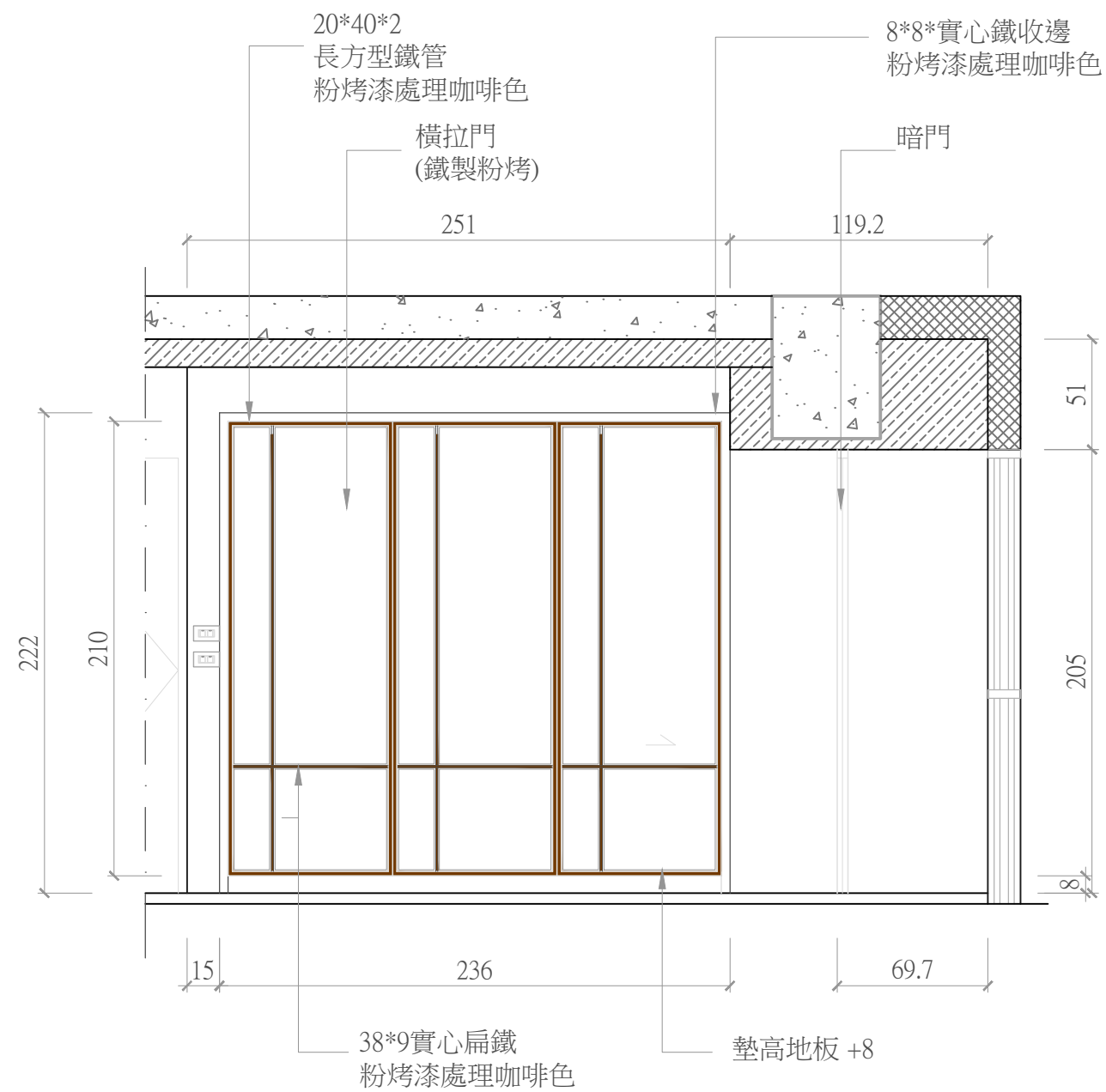
01 IE-05 客餐廳後向牆面立面圖
