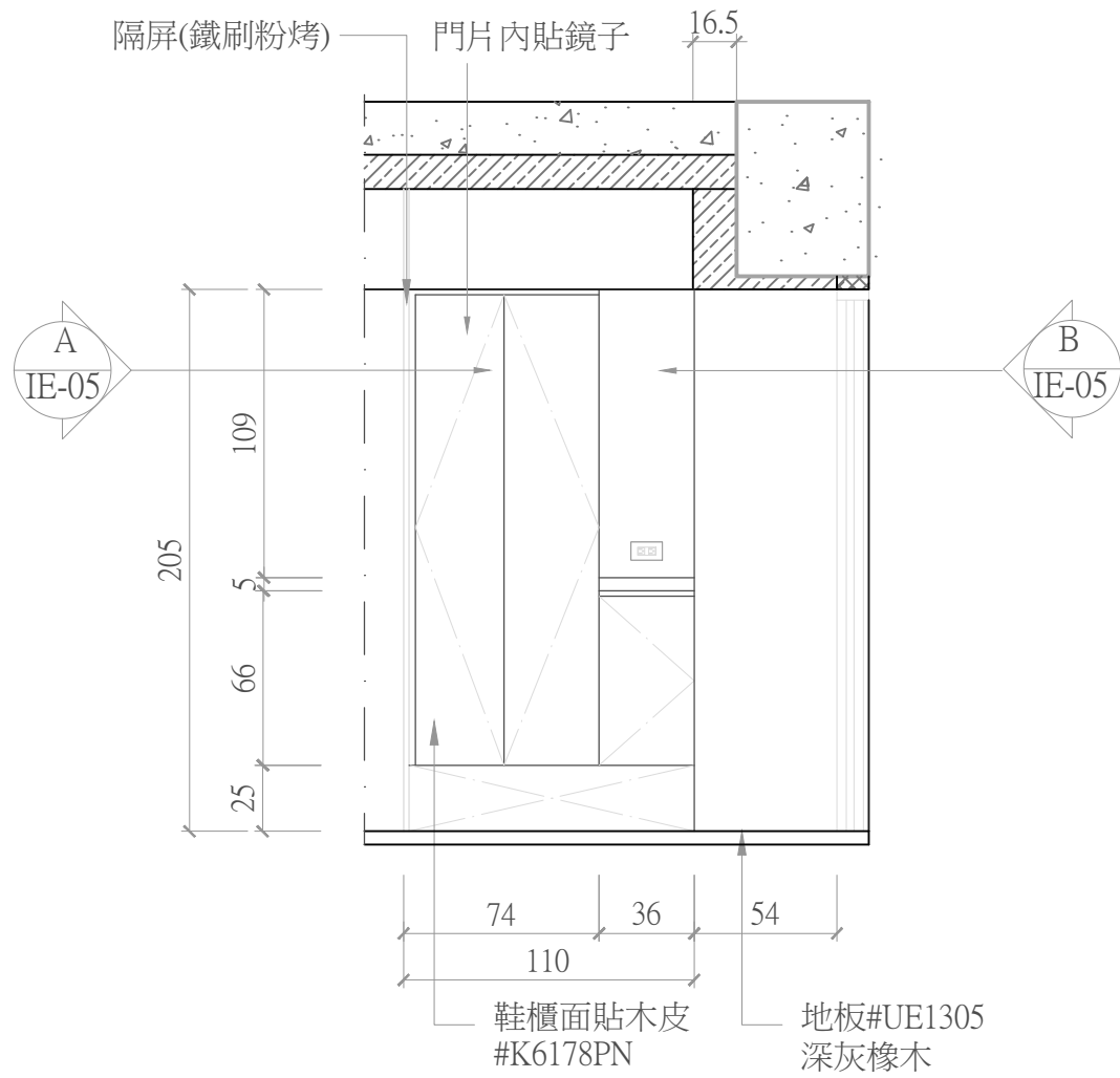
01 IE-05 客餐廳左向牆面立面圖
