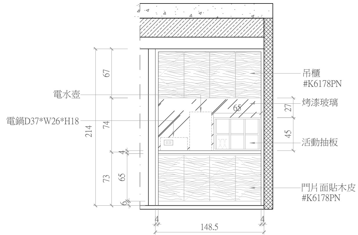
01 IE-04 置物高櫃立面圖
