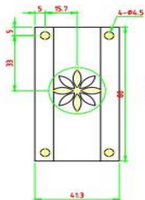
細部放大A 比例2:1
