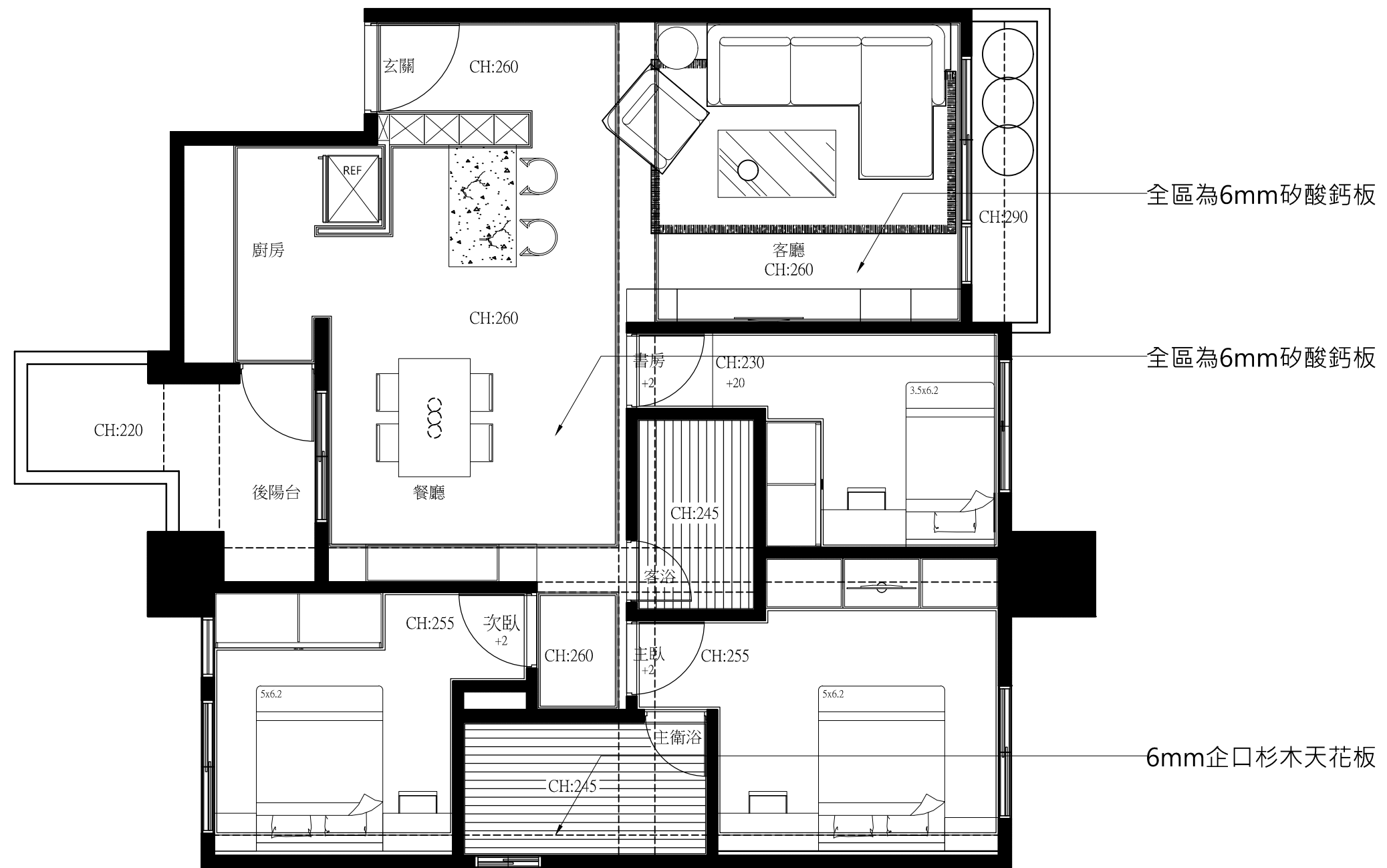
3 A 天花板圖 S:1:60 單位:cm
