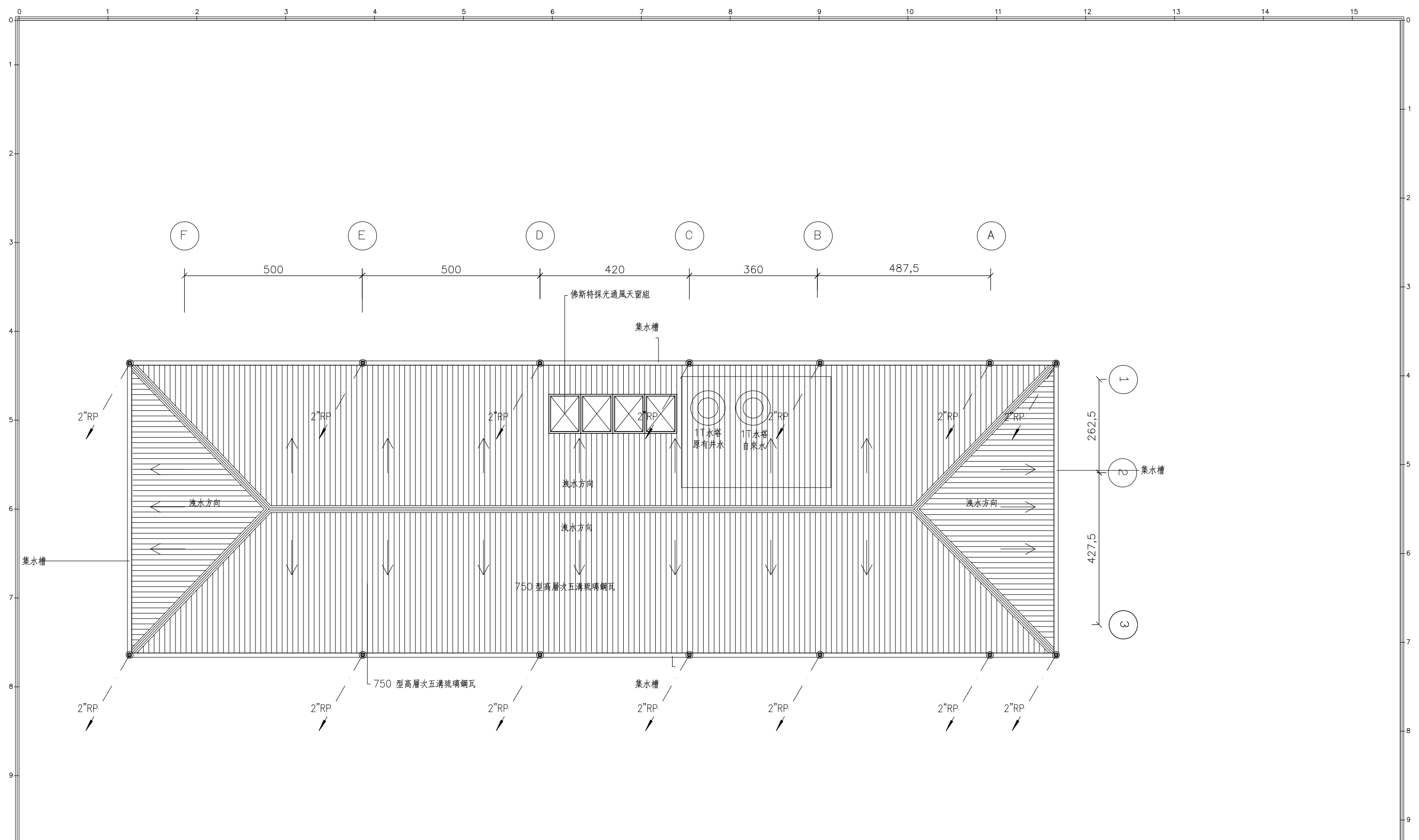
屋頂層平面圖 S:1/100(in A3)
