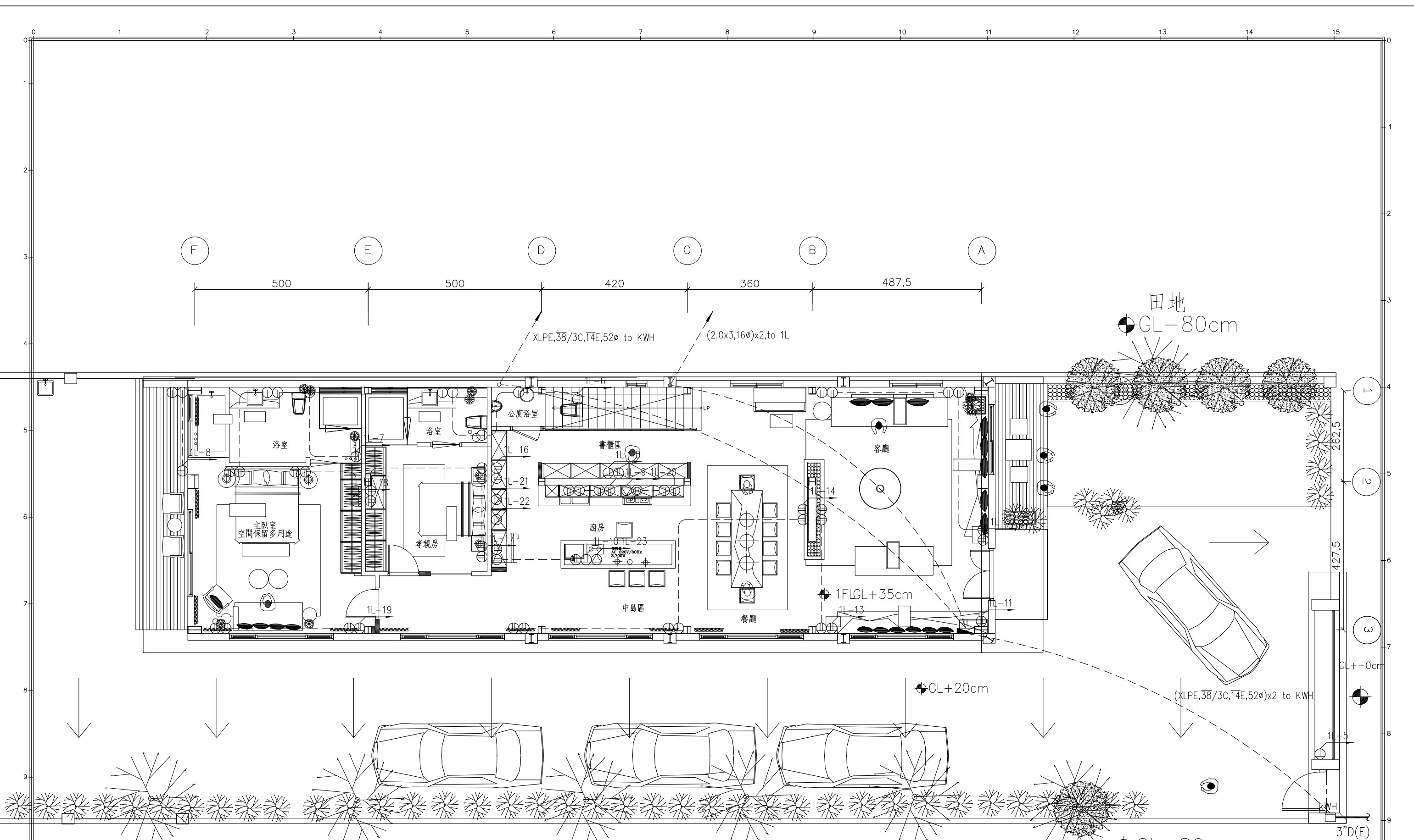
壹層平面圖 S: 1/100(in A3)
