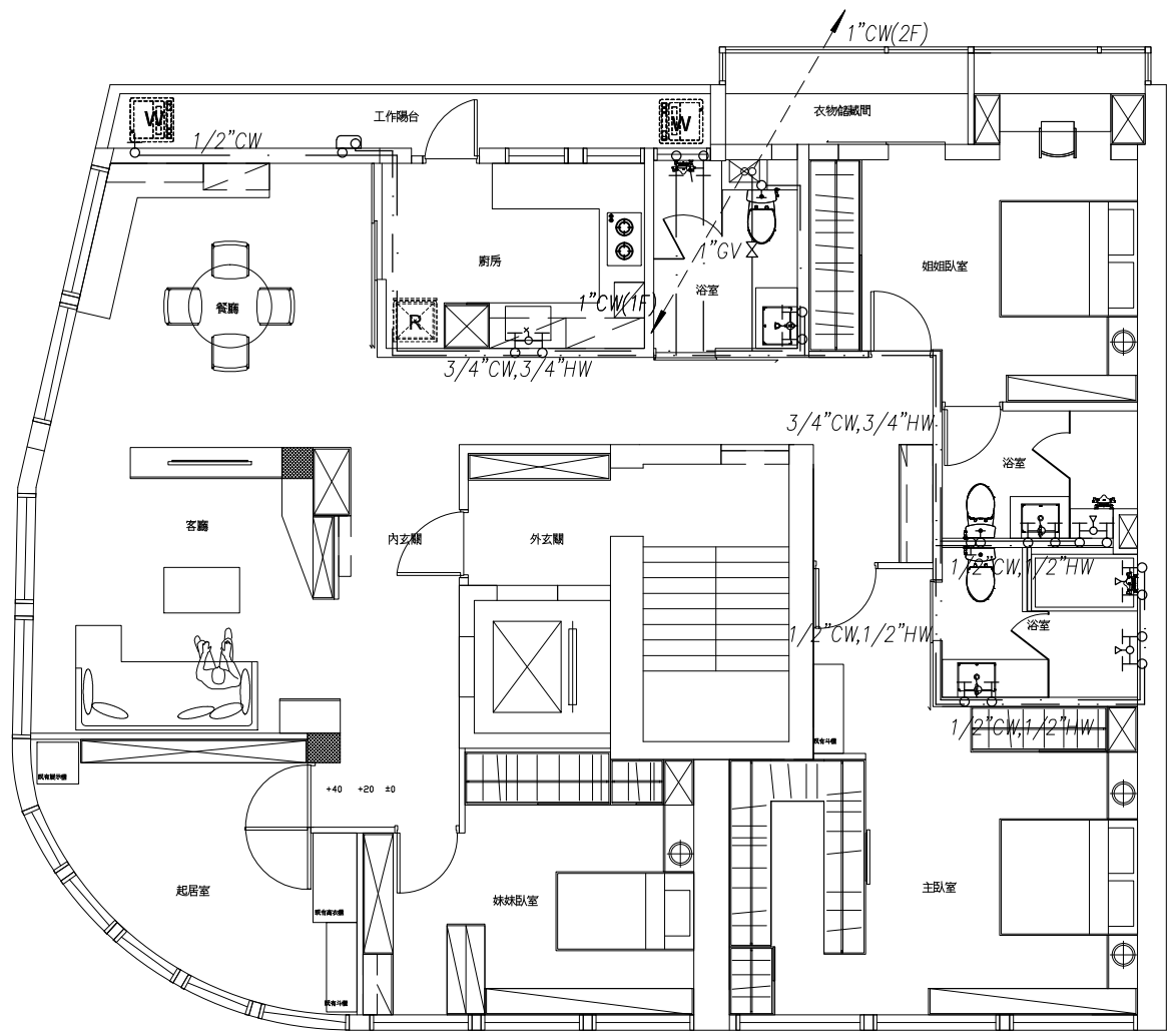
貳層平面圖 S:1/100(in A3)
