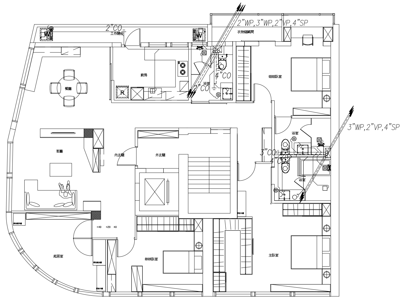
貳層平面圖 S:1/100(in A3)
