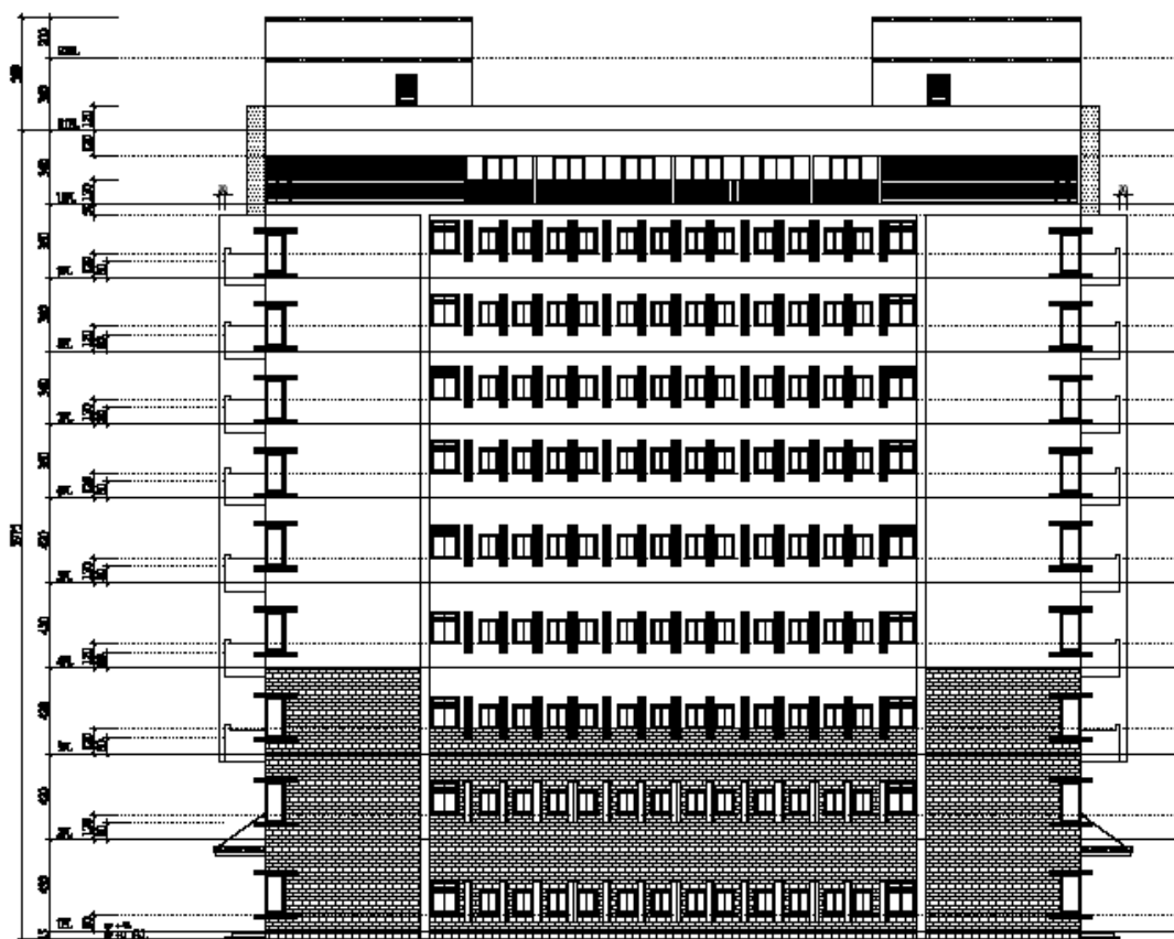
左側立面圖 S:1/200
