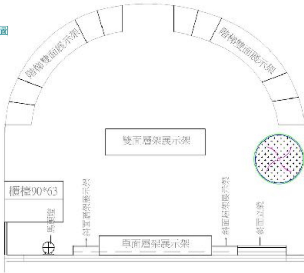
櫃位平面配置圖
