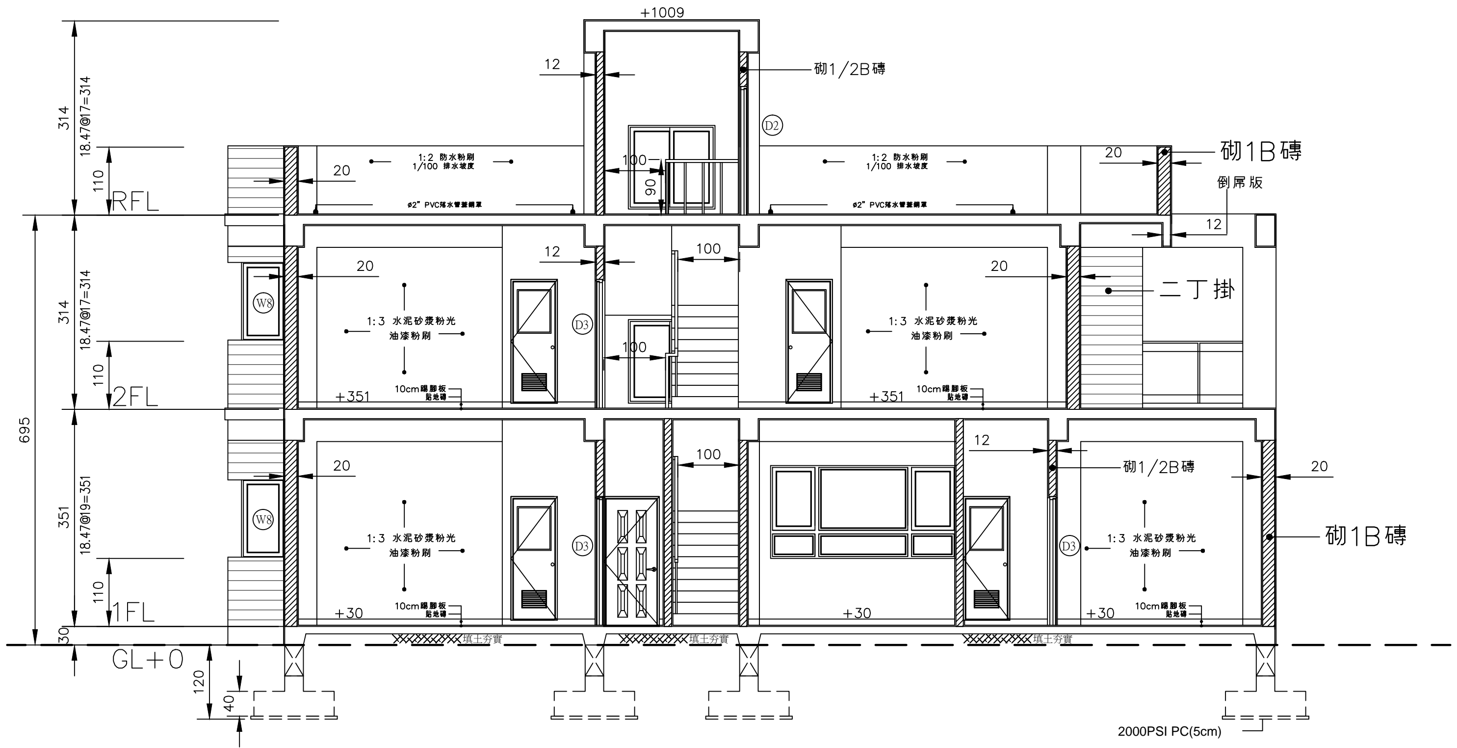
2/A3 剖面 S:1/60
