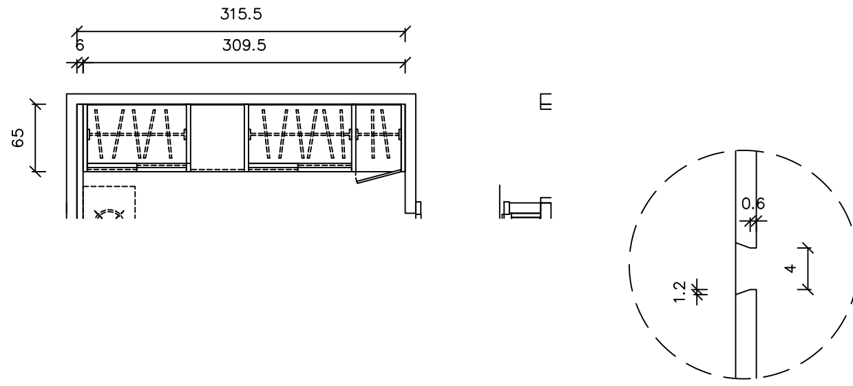
門片取手溝 詳圖三
