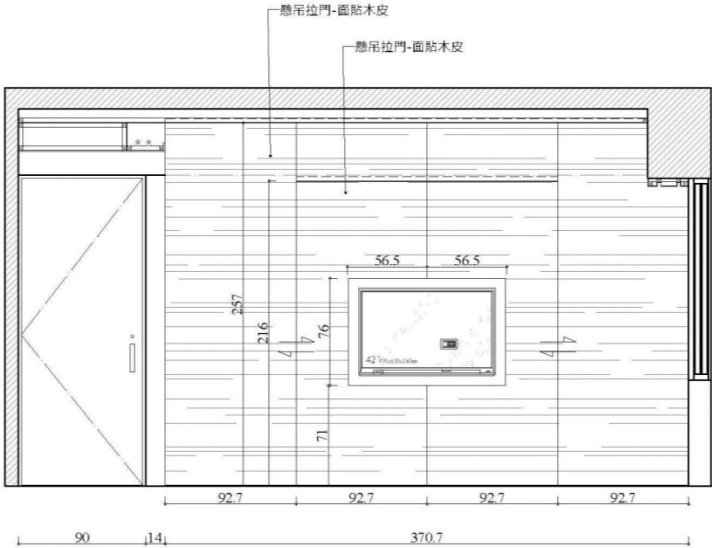
1 臥室立面圖 E-3 S=1/30 單位=CM
