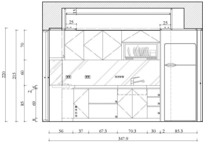
1 廚房立面圖 E-2 S=1/30 單位=CM
