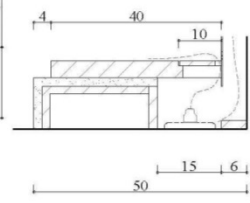
詳圖(一) S:1/10
