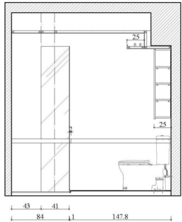
3 客浴立面圖 E-5 S=1/30 單位=CM
