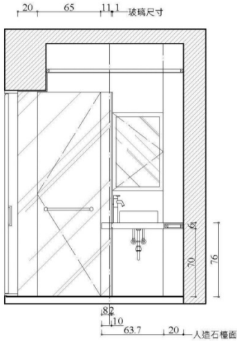
4 客浴立面圖 E-5 S=1/30 單位=CM
