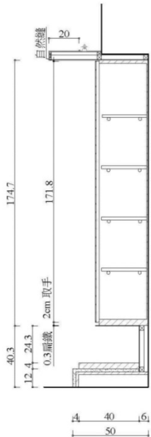
A-A' 剖面圖 S:1/20
