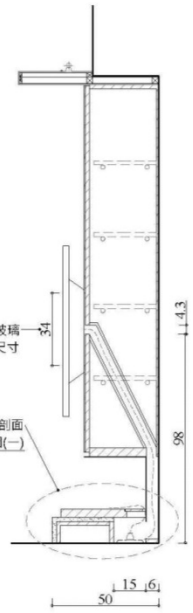
B-B' 剖面圖 S:1/20
