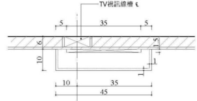
詳圖(二) S:1/10
