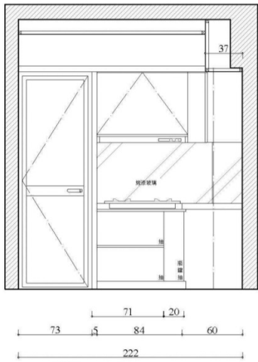
2 廚房立面圖 E-2 S=1/30 單位=CM
