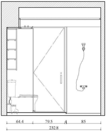
1 客浴立面圖 E-5 S=1/30 單位=CM
