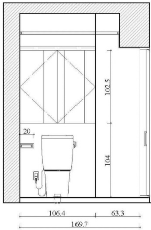
2 客浴立面圖 E-5 S=1/30 單位=CM
