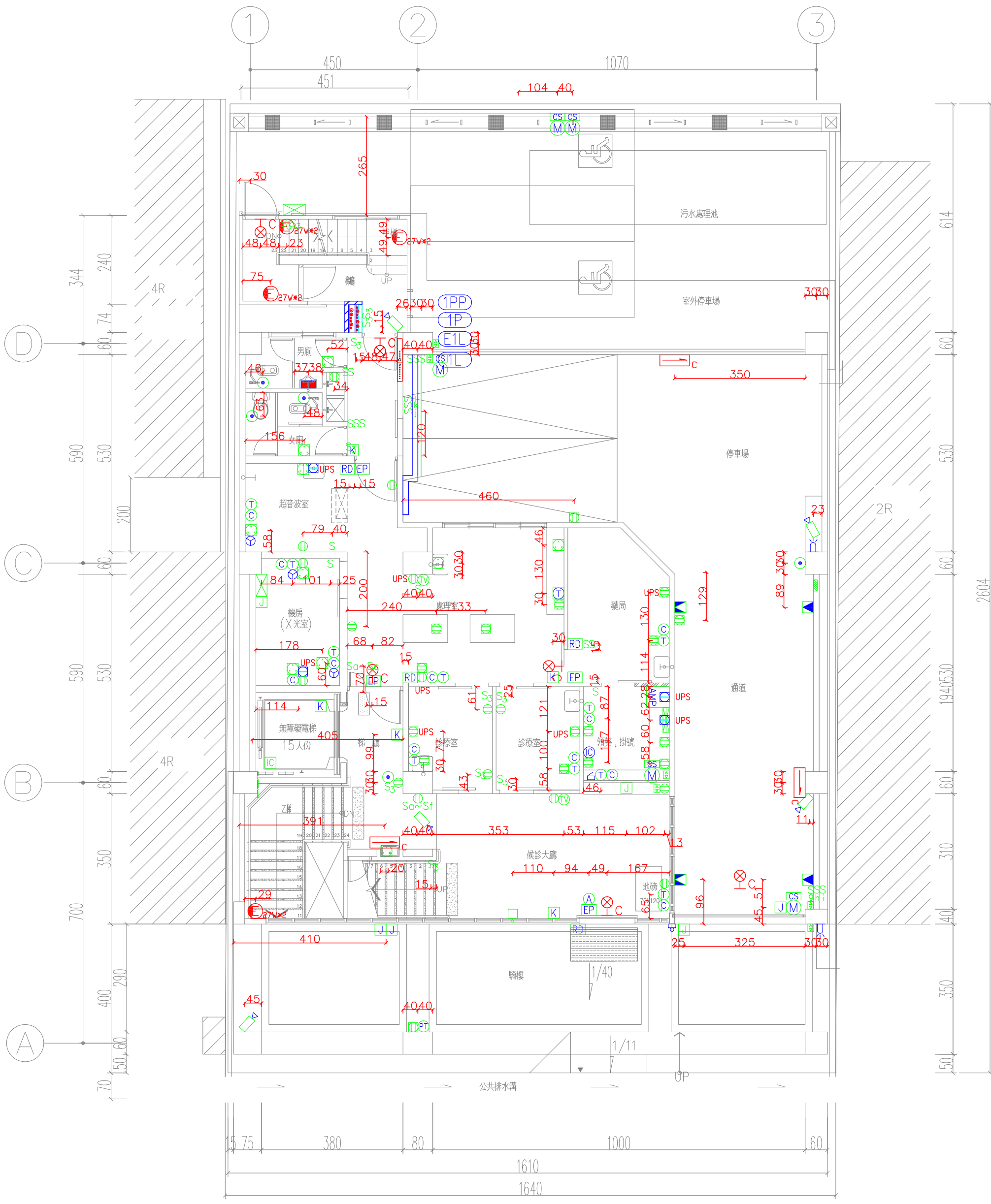
壹層平面圖
