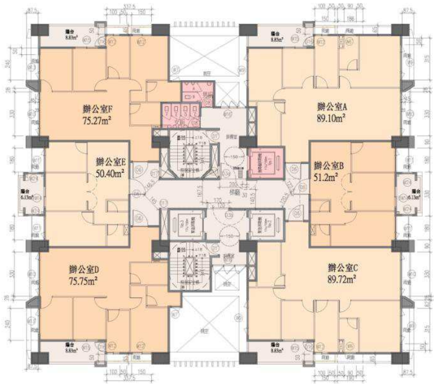
■ 標準層平面圖
