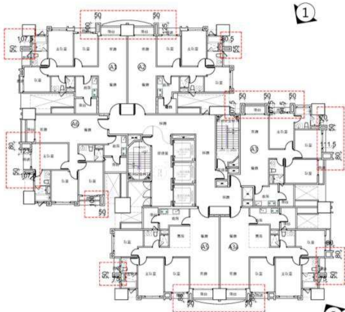
A棟-標準層平面圖
