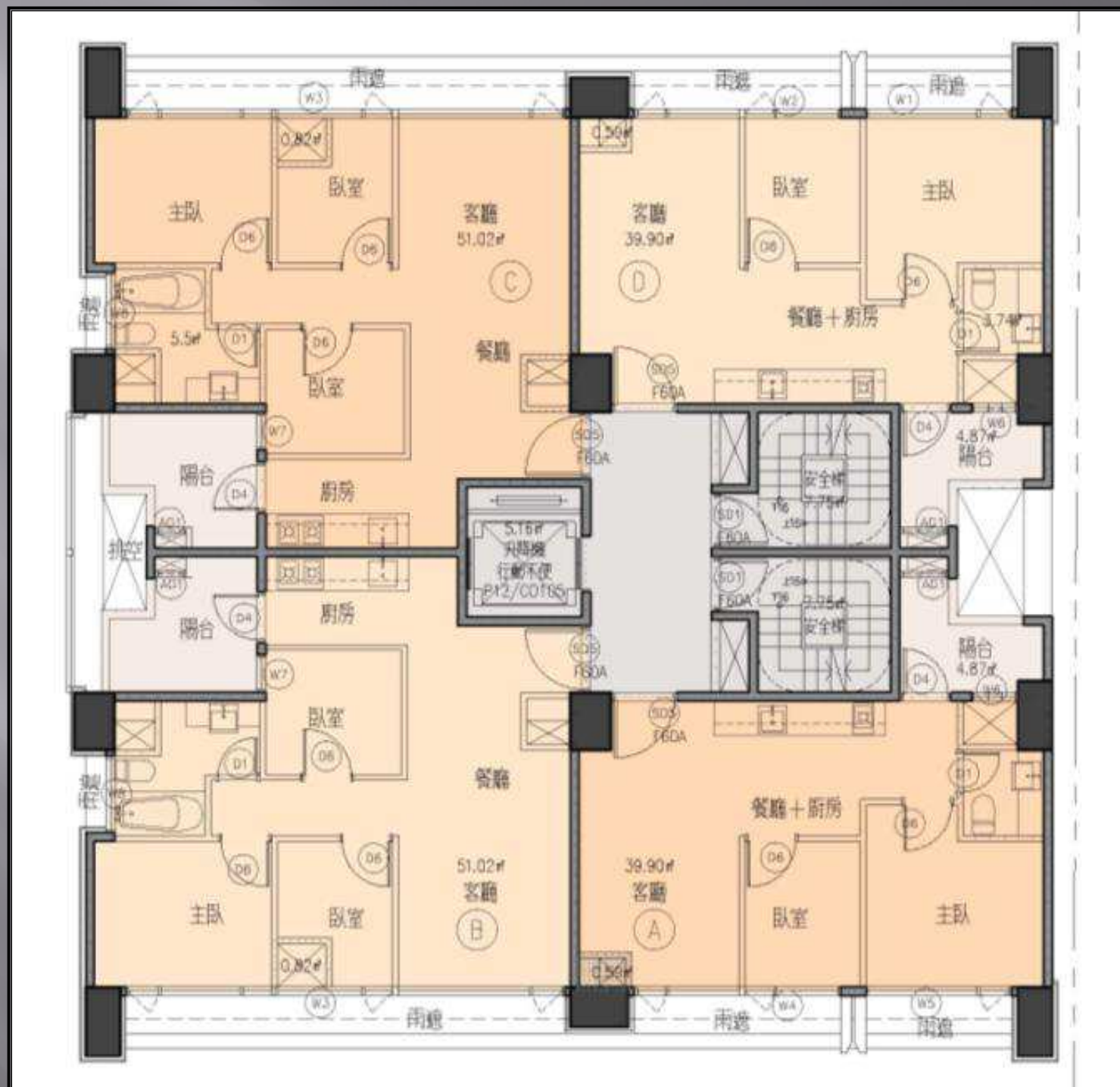
■ 標準層平面圖
